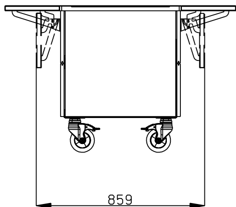
Bočna/o
